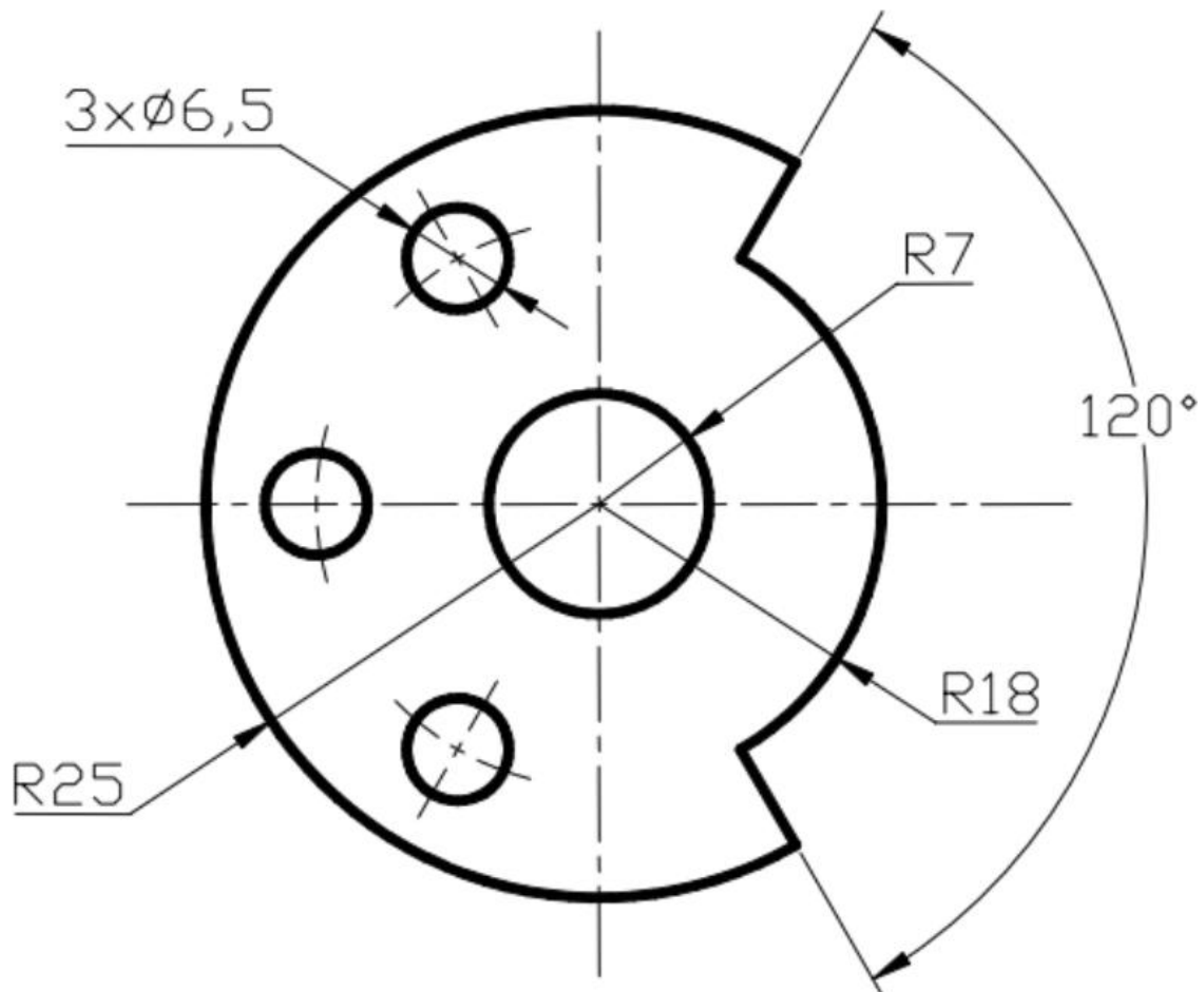
Рисунок 1.2 – Кресленик завдання
